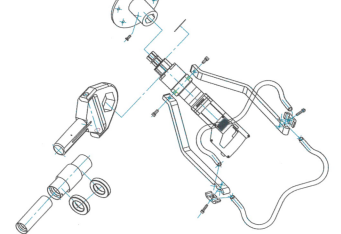
分解図
